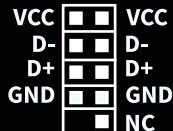
Conector USB 2.0 da Placa-Mãe
